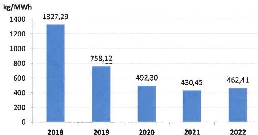
Wielkość emisji CO 2 do powietrza w przeliczeniu na MWh wytworzonej energii elektrycznej, w okresie od 2018 do 2022 roku
