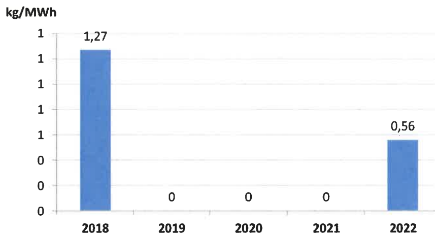
Wielkość emisji SO 2 do powietrza w przeliczeniu na MWh wytworzonej energii elektrycznej, w okresie od 2018 do 2022 roku
