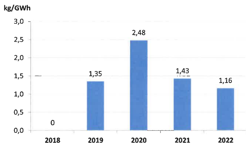
Wielkość emisji pyłów do powietrza w przeliczeniu na GWh wytworzonej energii elektrycznej, w okresie od 2018 do 2022 roku
