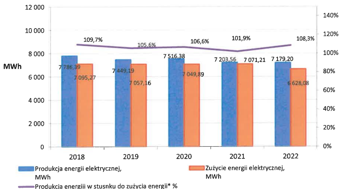
Bilans energii elektrycznej RCGW S.A w MWh/rok
