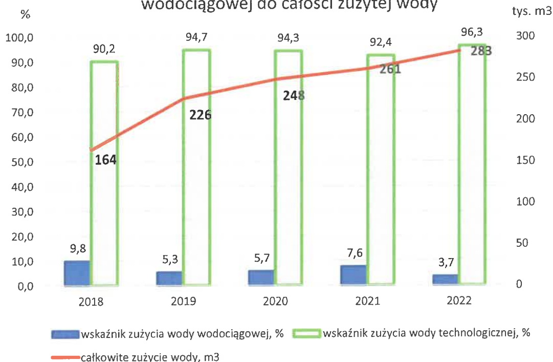
Wskaźnik % udziału zużycia wody technologicznej i wodociągowej do całości zużytej wody
